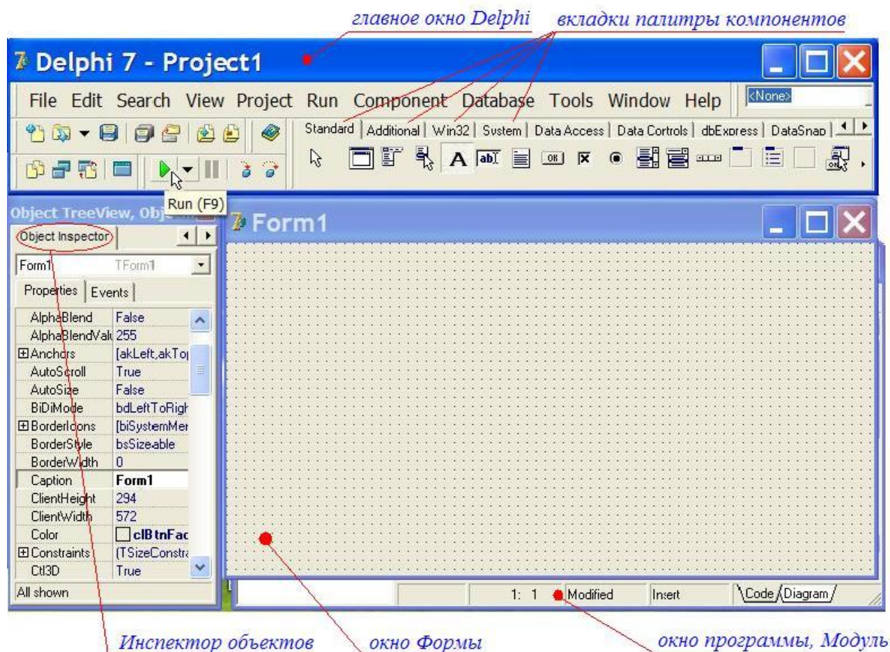
Рис. 1. Окна Delphi
