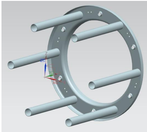
Рис. 26. 3D модель камеры сгорания малоразмерного ГТД (часть 2)
