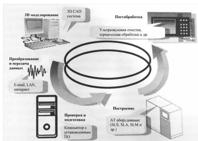
Рис. 4. Технологический процесс СЛС
