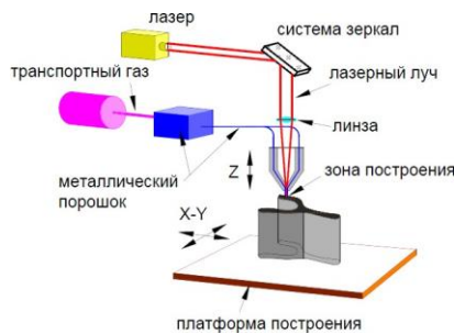
Рис. 1. Непосредственное нанесение порошка
