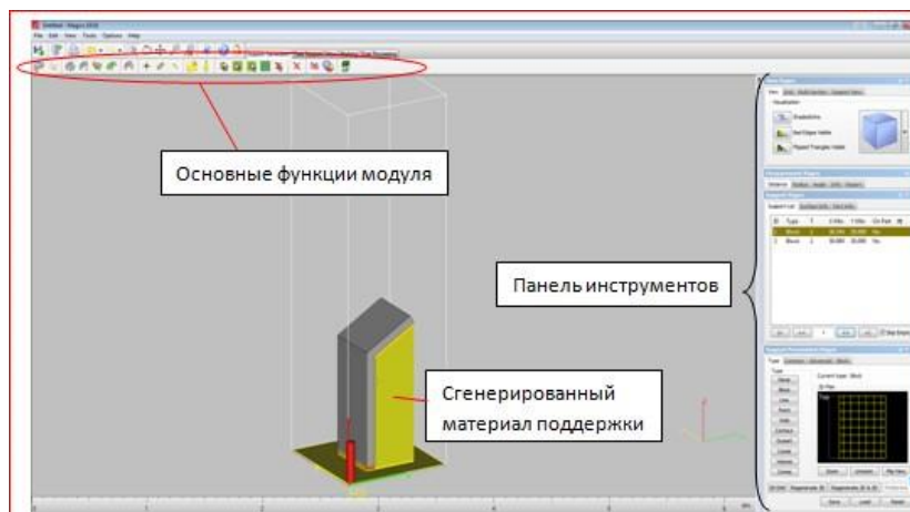
Рис. 16. Материал поддержки и основные элементы модуля
