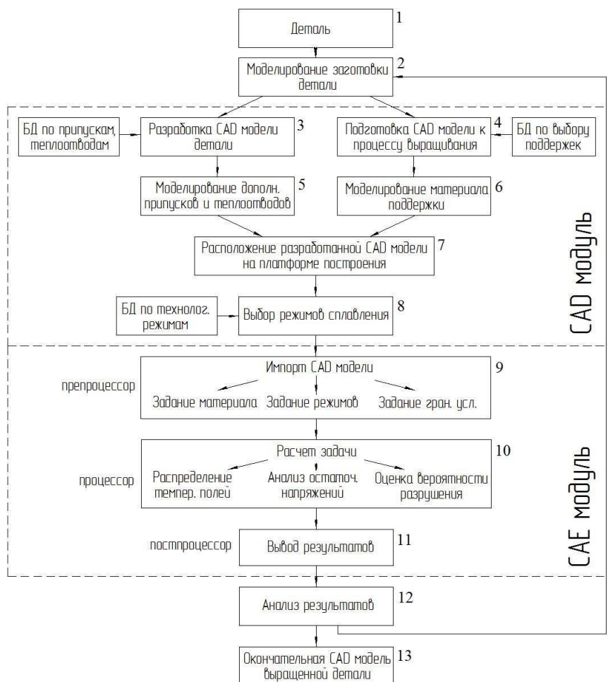
Рис. 6. Алгоритм разработки ТП СЛС
