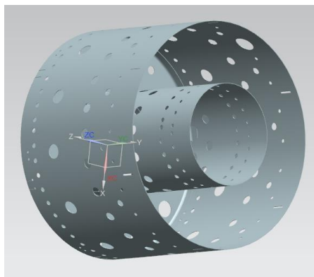
Рис. 25. 3D модель камеры сгорания малоразмерного ГТД (часть 1)
