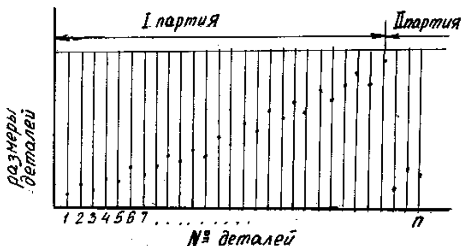
Рис. 3. Точечная диаграмма
