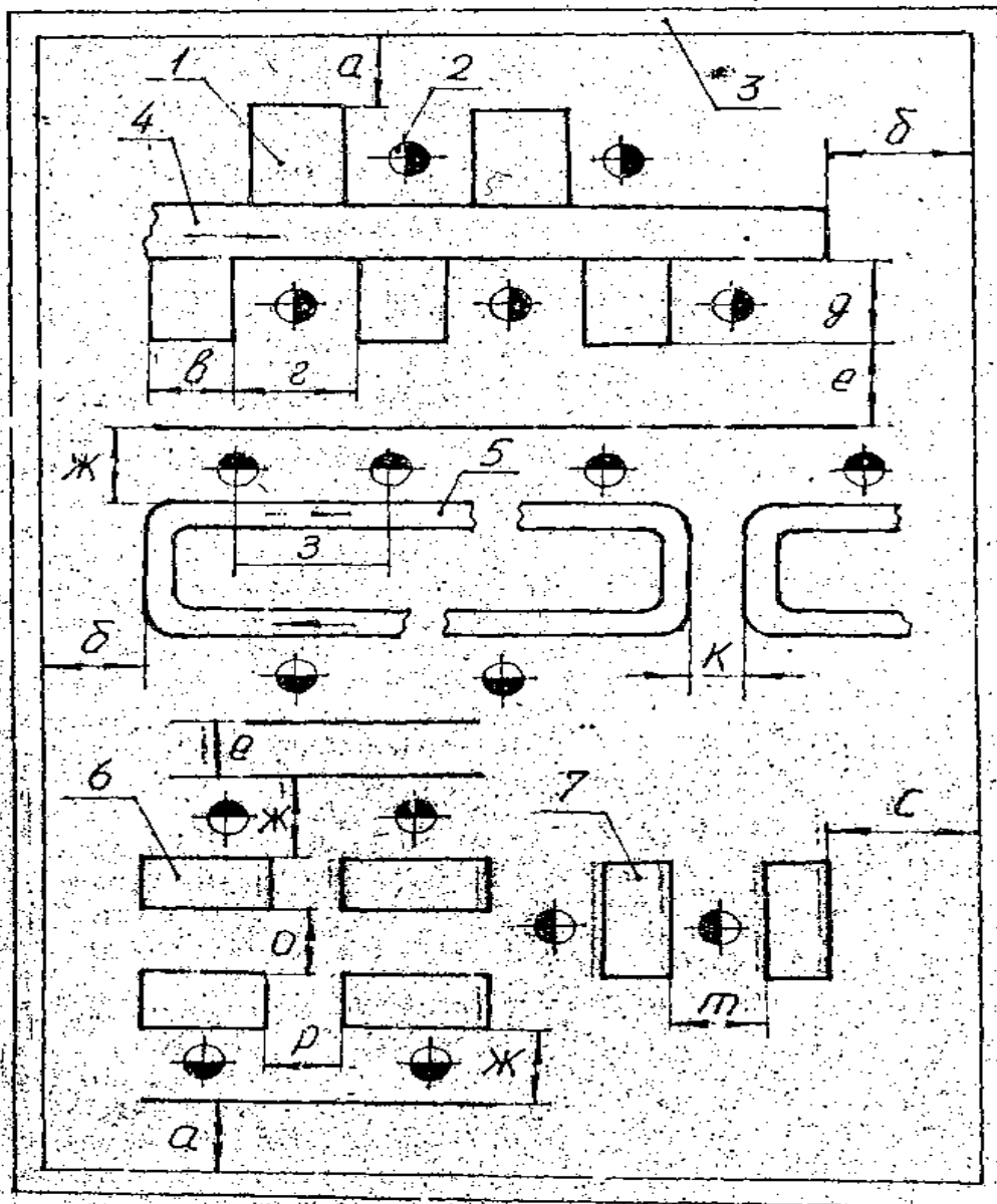
Рис.3. Нормативные расстояния между технологическим оборудованием
