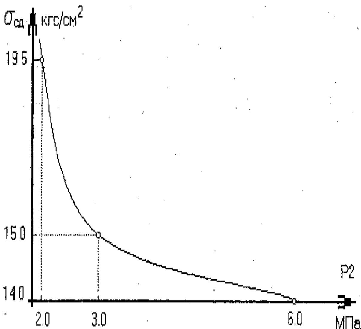
Рис. 5. Зависимость прочности на сдвиг от уровня высокого давления
