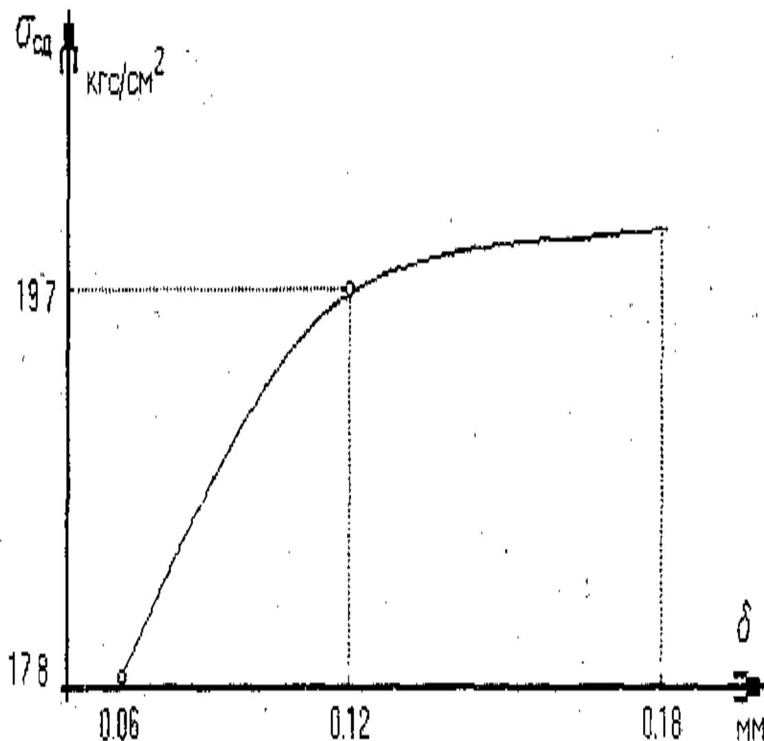
Рис. 3. Зависимость прочность на сдвиг от толщины прокладки между слоями
