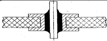
Скелетная форма. Галтели вогнутые
