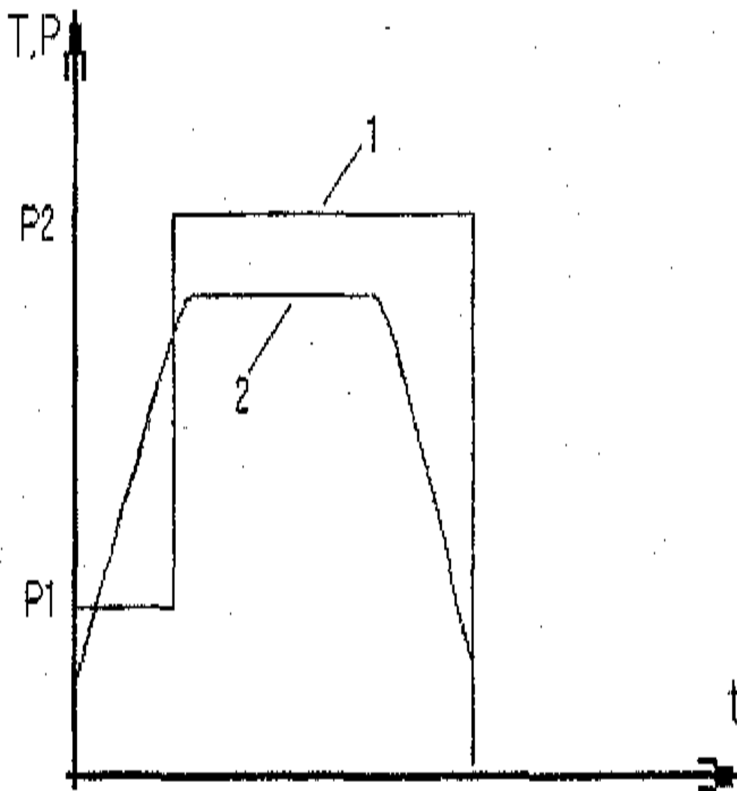
Рис. 4. Характер изменения давления (1) и температуры (2) при прессовании МПП
