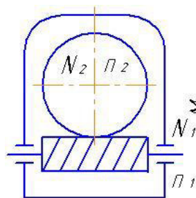
Рис. 4 Схема редуктора
