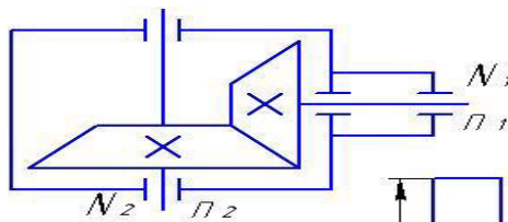
Рис. 2 Схема редуктора
