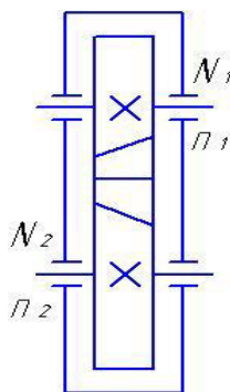
Рис. 3 Схема редуктора
